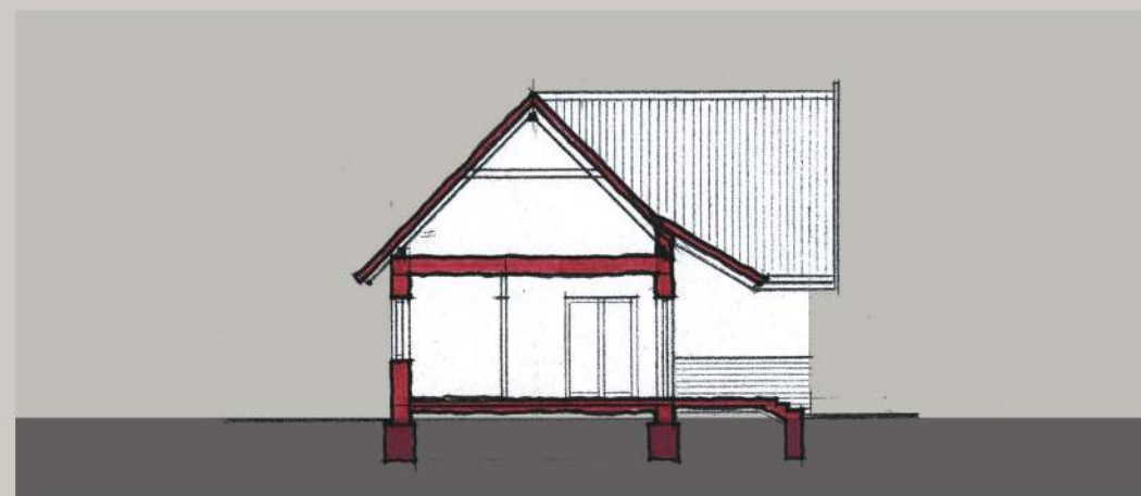
metszet m=1:200
