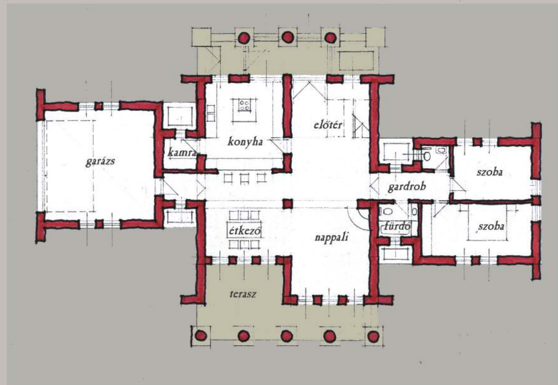
földszinti alaprajz m=1:200
