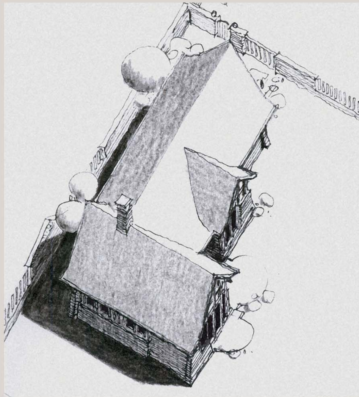
távlati kép m=1:200
