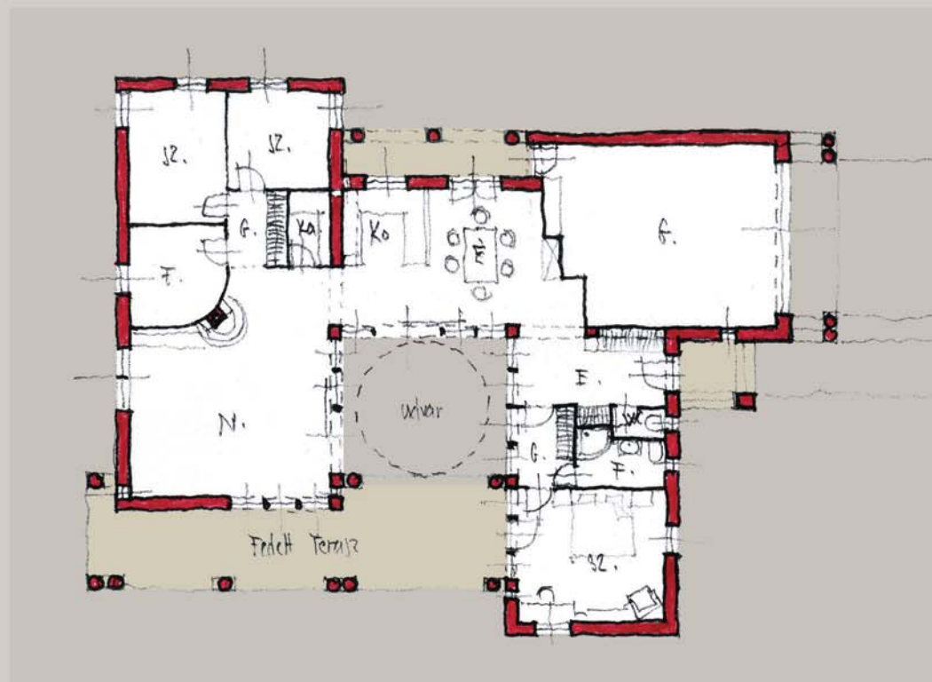
alaprajz m=1:200
